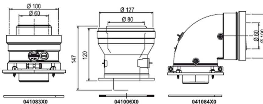
21. ábra – Koncentrikus induló idomok
