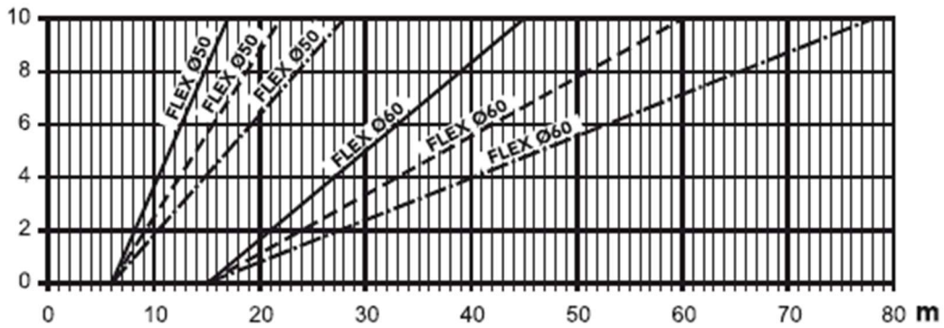
25. ábra – Füstgázvezeték paraméterek
